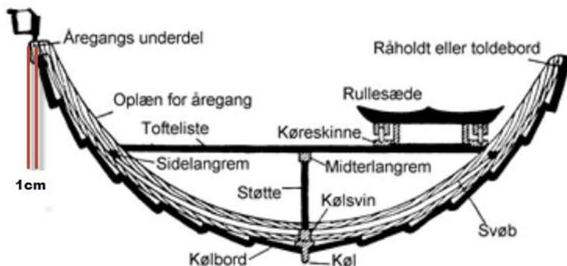
Figur 6 - fra Langtursstyrmandsbogen 2020-2021
